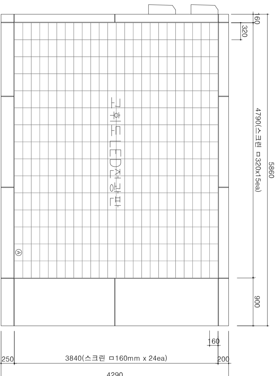
1 정면도 SCALE: 1/60
