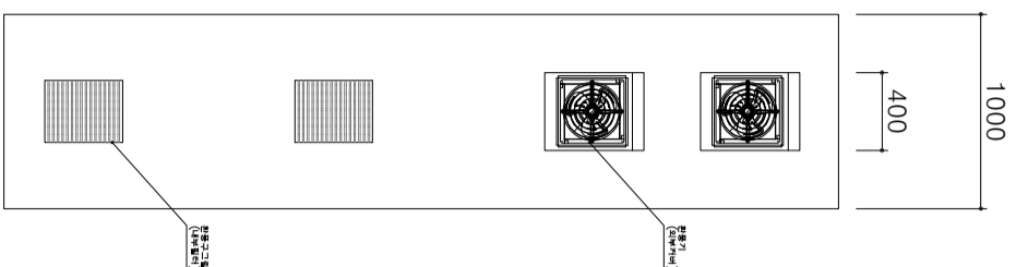
1 좌측면도 SCALE: 1/60
